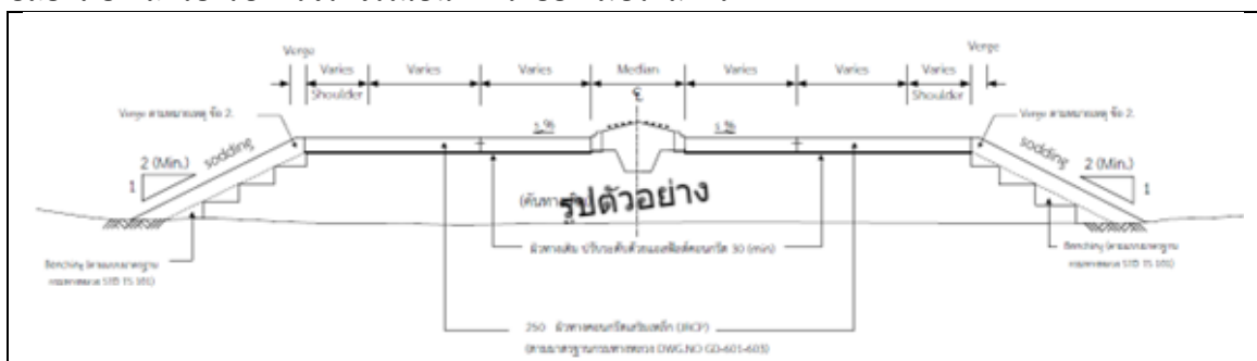
ที่มา : การเสริมผิวทางเดิมด้วยผิวทางคอนกรีตเสริมเหล็ก คูขวโรจน์, จุฬา สุนิตย์สกุล, สำนักวิเคราะห์และตรวจสอบ กรมทางหลวง
