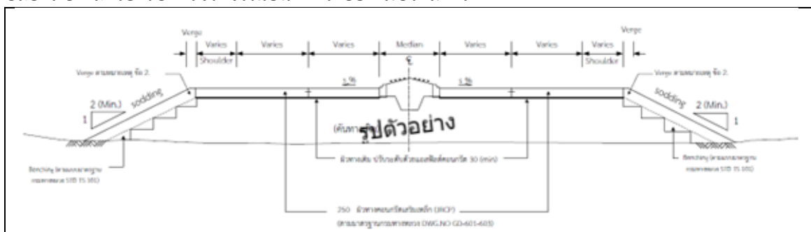
ที่มา : การเสริมผิวทางเดิมด้วยผิวทางคอนกรีต, ชัยรัตน์ ศุภชวโรจน์, จุฬา สุณิตยสกุล, สำนักวิเคราะห์และตรวจสอบ กรมทางหลวง
