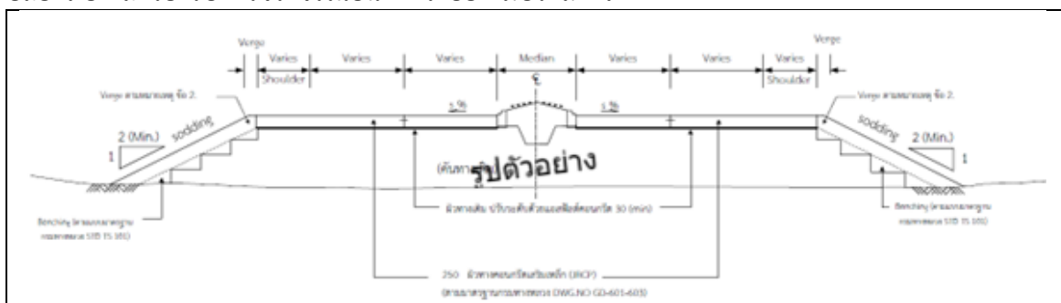
ที่มา : การเสริมผิวทางเดิมด้วยผิวทางคอนกรีต, ชัยรัตน์ ศุภชวโรจน์, จุฬา สุณิทยสกุล, สำนักวิเคราะห์และตรวจสอบ กรมทางหลวง
