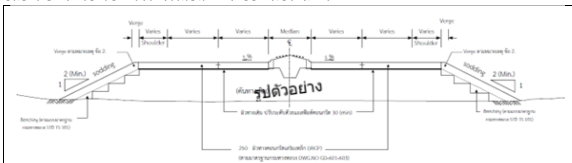
ที่มา : การเสริมผิวทางเดิมด้วยผิวทางคอนกรีต, ชัยรัตน์ ศุภขวโรจน์, จุฬา สุนิตยสกุล, สำนักวิเคราะห์และตรวจสอบ กรมทางหลวง
